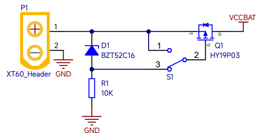
电源接口/开关
