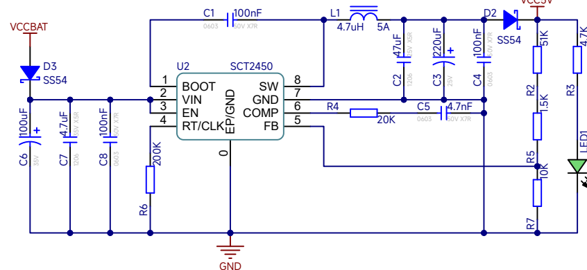
5V电源
