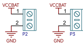
电机电源接口
